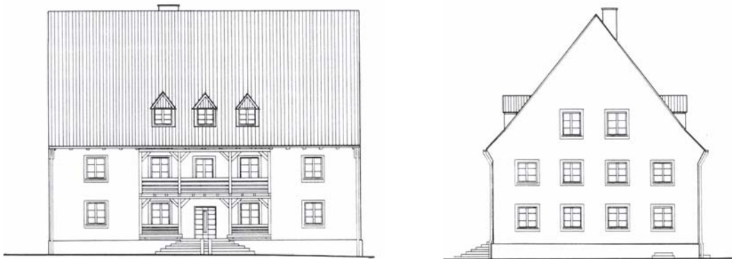
Ansichten
