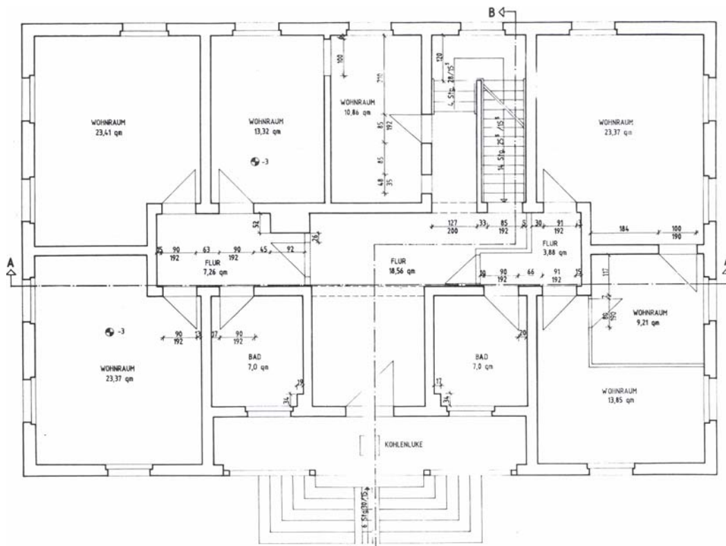
Grundriss Erdgeschoss
